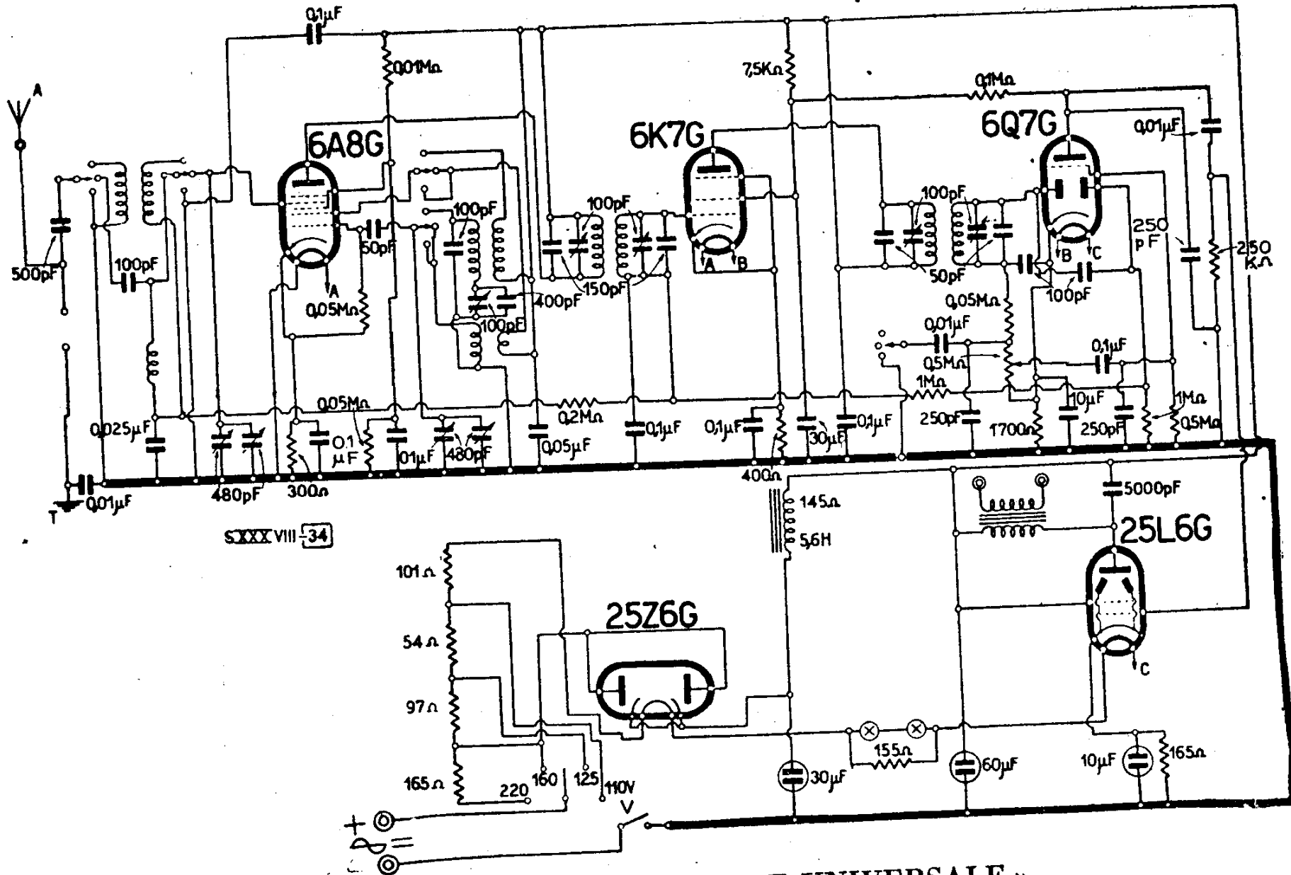
WATT RADIO - MOD. « ALFIERE UNIVERSALE »
